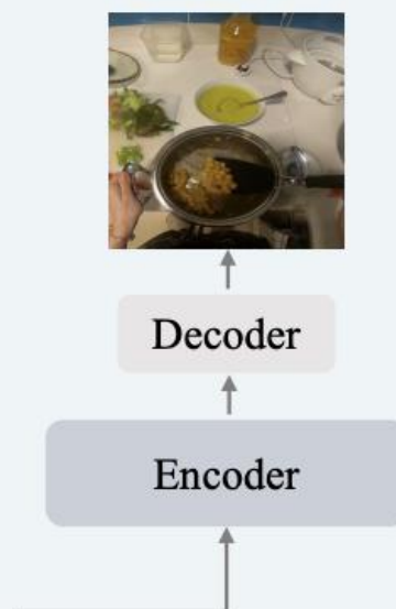
(b) Autoencoder
